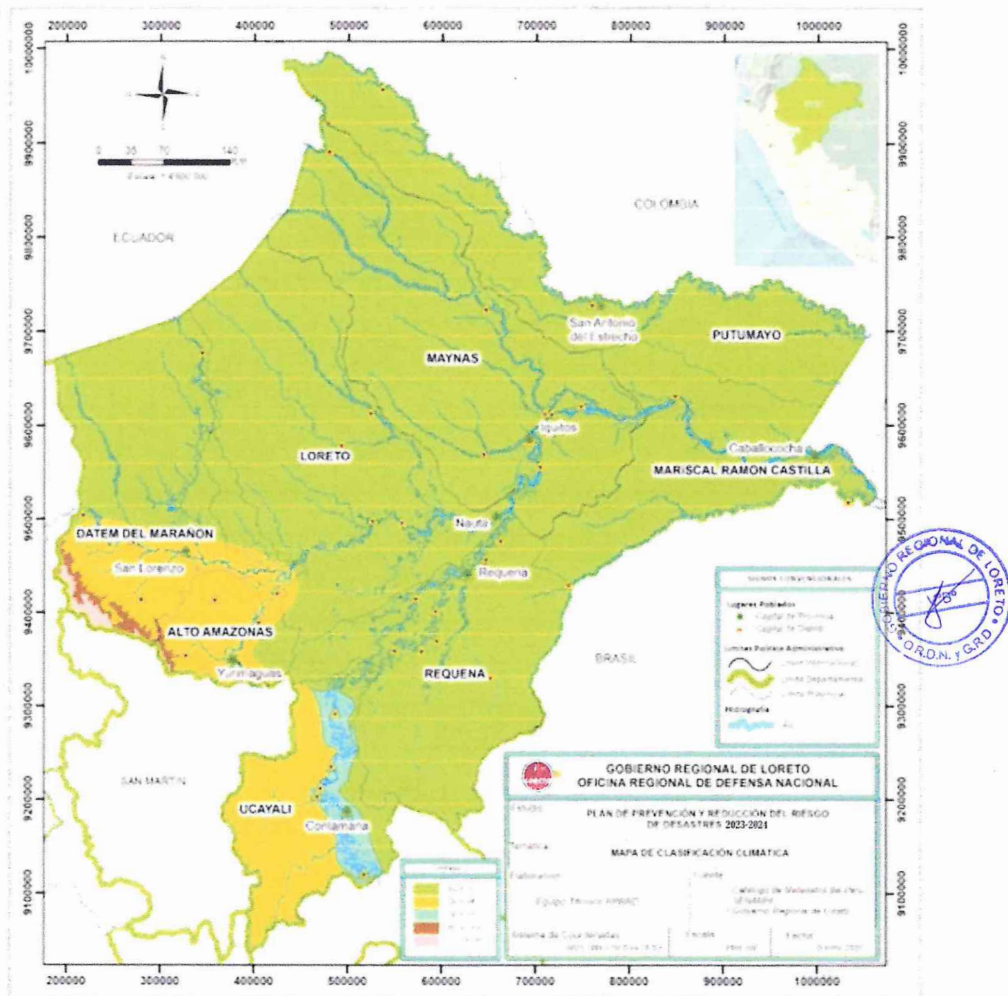
Ilustración 37: Mapa de clasificación climática
